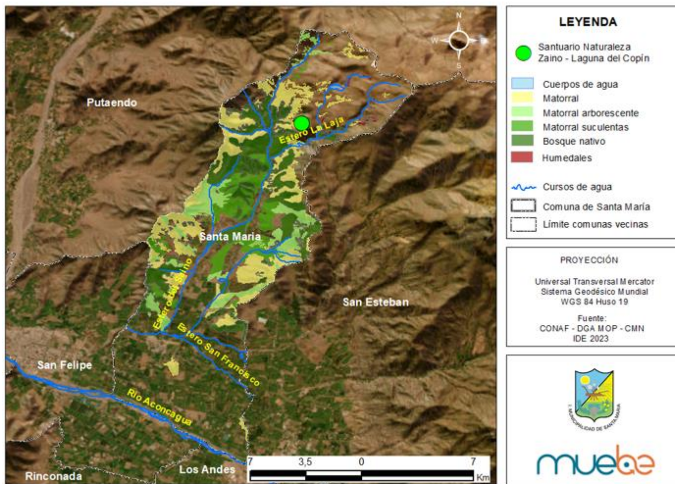
Ilustración 7. Principales unidades vegetacionales y ambientales en la comuna de Santa María
