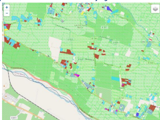
Ilustración 20. Representación de usos de suelo en fragmento de la comuna de Santa María
