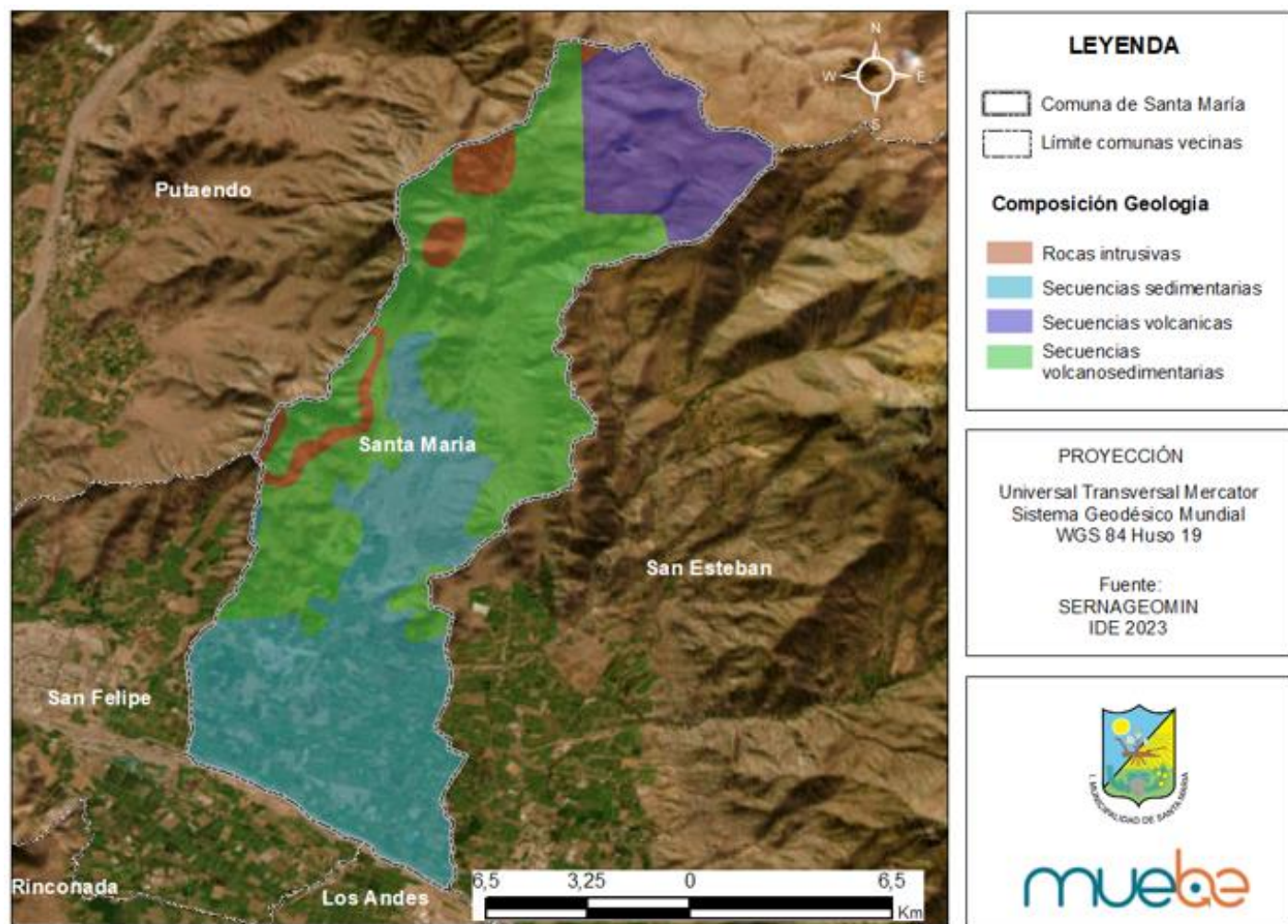
Ilustración 3. Composición geológica de la comuna de Santa María
